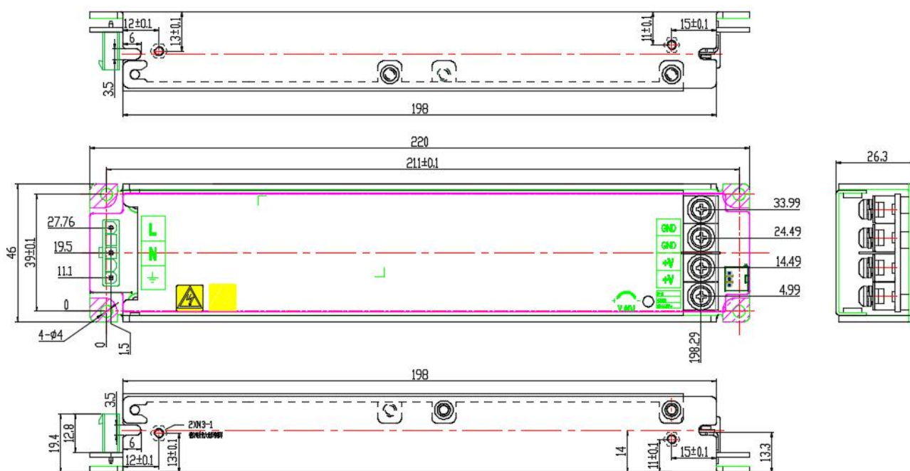
外形尺寸及安装孔——端子坐标图
